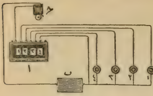
( جهاز [ مرکب ] )
